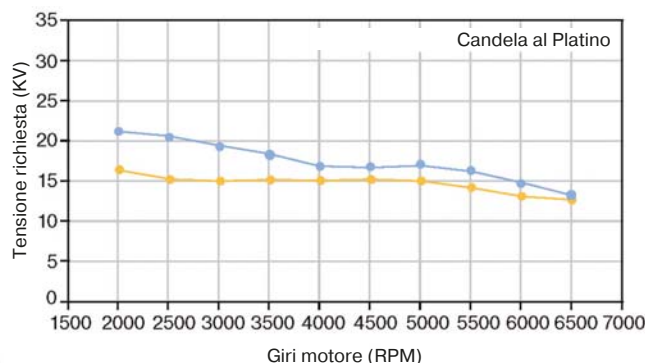
La tensione richiesta per l'accensione aumenta nei motori alimentati a gas.
