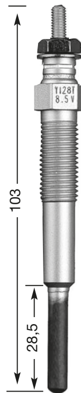
Y-128 T M 10 x 1.25 12 Hex 8,5 V
