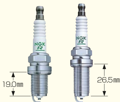
Candela con filettatura estesa Esempio: LFR5A-11
