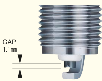
Gap maggiorato Esempio: BKR5E-11
