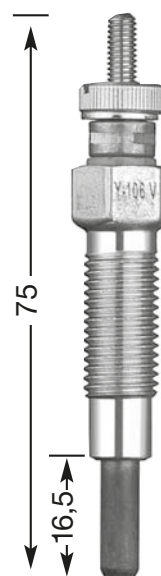
Y-106 V M 10 x 1.25 12 Hex 10,5 V
