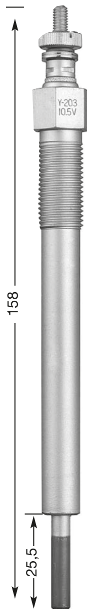
Y-203 M 12 x 1.25 14 Hex 10,5 V
