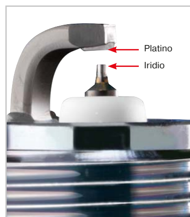
Elettrodo centrale con riporto in lega all'Iridio ed elettrodo di massa con riporto in lega al Platino, entrambi saldati al laser: accensioni sicure e il massimo della resistenza per tutta la durata di esercizio.
