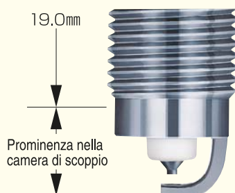
Corpo metallico esteso Esempio: BKR6EPA-8
